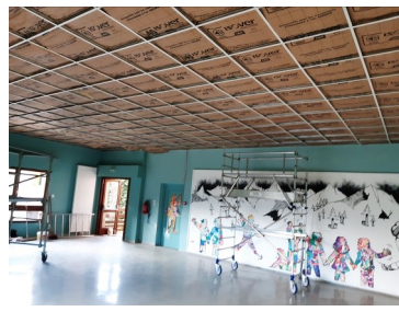
Montage des structures et pose de l'isolant thermique
